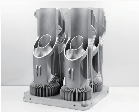
样品名称：智能水下机器人散热器 打印设备：FS301M-2 打印材料：铝合金
